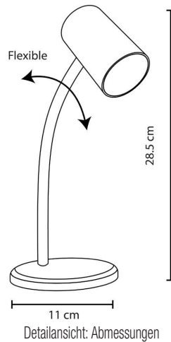
Detailsicht: Abmessungen
