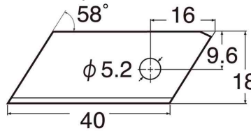
Ersatzklinge BZL11P, Detailsicht
