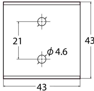
Ersatzklinge BKT-300P, Detailsicht
