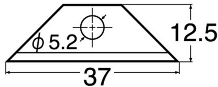
Ersatzklinge BR-400P, Detailsicht
