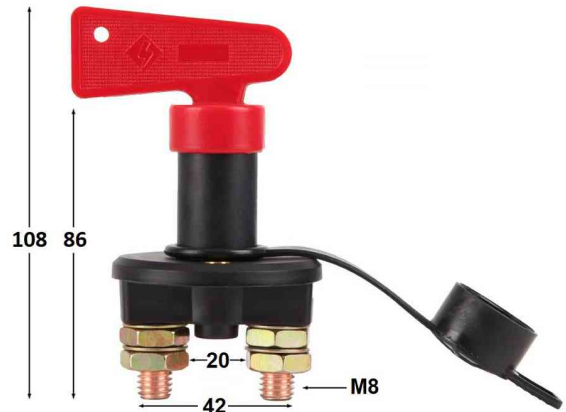
Batterie-Trennschalter, 100 A
