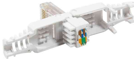
RJ45-Steckverbinder Kat.6, UTP, werkzeuglos
